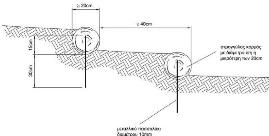
Εικόνα 11: Δημιουργία βαθμίδων με χρήση εγκάρσιων κορμών καστανιάς
