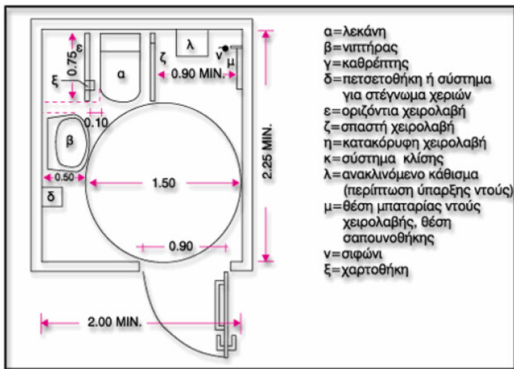
Σχήμα 3: Τυπική κάτοψη του χώρου W.C. ΑμεΑ.
