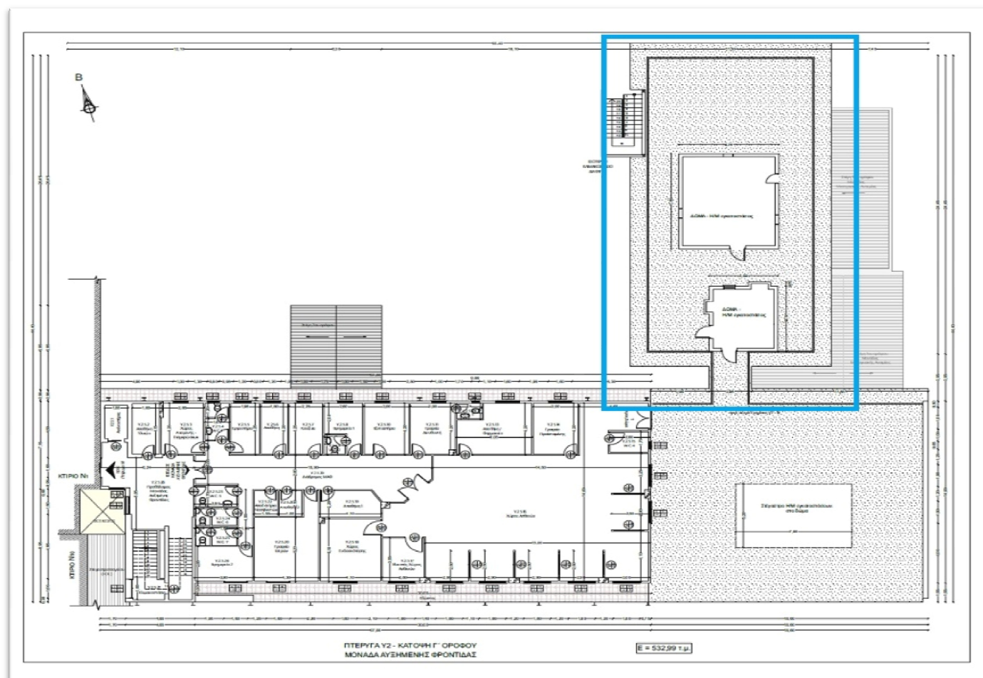
Σχέδιο 1. Κάτοψη δώματος Υ2 Κτιρίου πάνω από την Ουρολογική Κλινική
